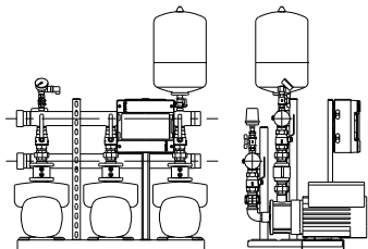
Slika 9 Hydro Multi-E s jednofaznim CME crpkama
