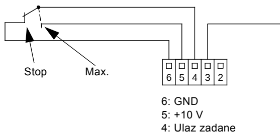
Slika 11 Spajanje tlačnih sklopki
