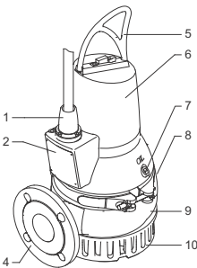
Slika 10 DP 10.65 crpka
