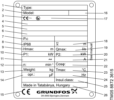
Slika 12 Natpisna pločica
