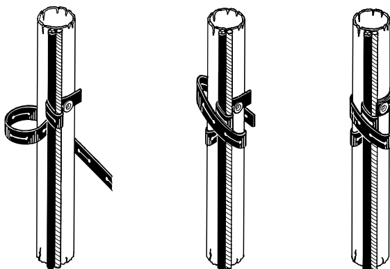
Slika 22 Postavljanje kabelskih vezica
